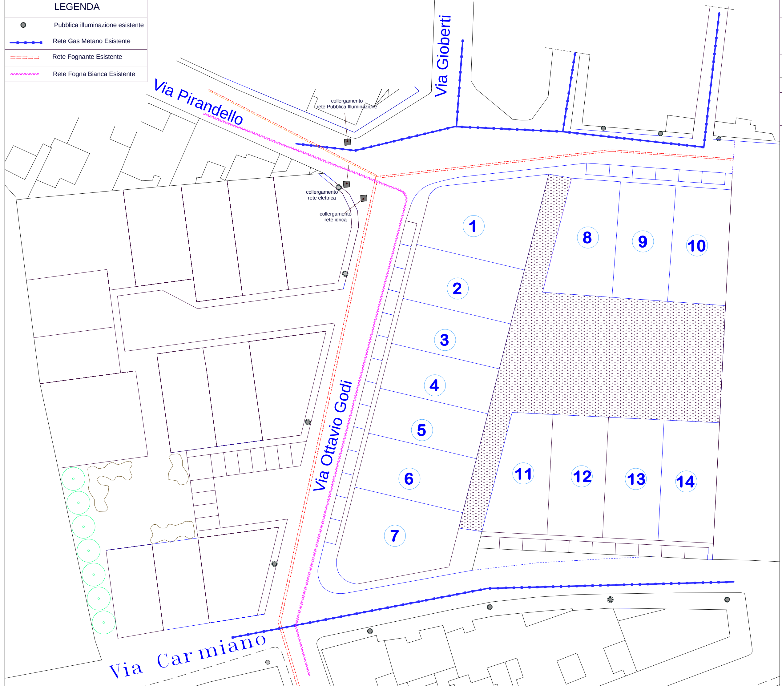
PLANIMETRIA - RETI IMPIANTI URBANIZZAZIONE PRIMARIA ESISTENTI
