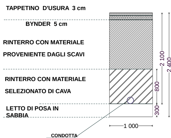
PARTICOLARE SEZIONE SCAVO AQP
