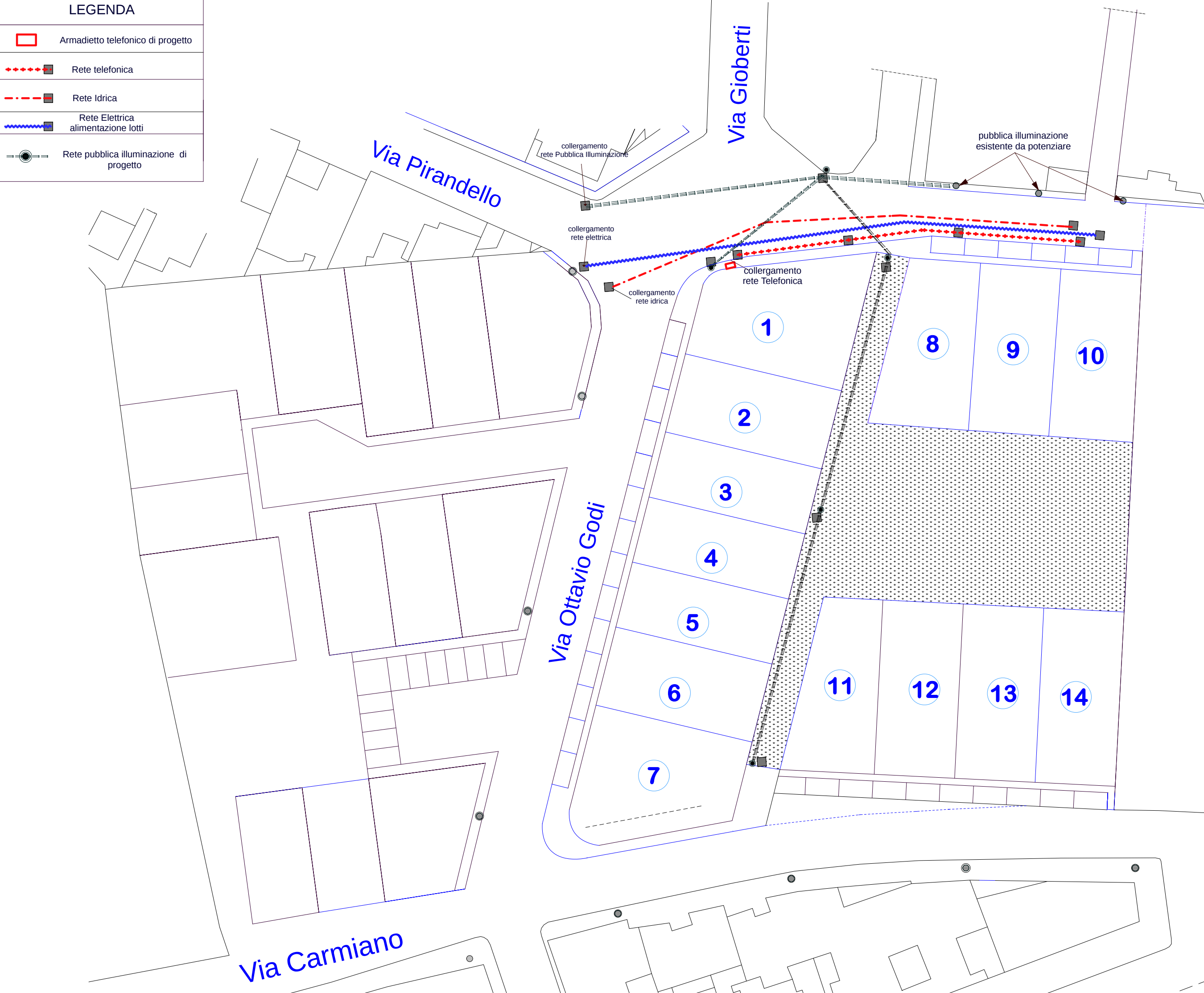
PLANIMETRIA - RETI IMPIANTI URBANIZZAZIONE PRIMARIA DI PROGETTO
